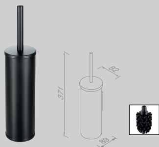
Toiletborstel met houder (Zwarte borstelkop) Toilet brush and holder (Black brush head) 916511-66
