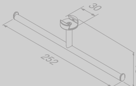
Toiletrolhouder zonder klep dubbel (Chrome) Toilet roll holder without cover double (Chrome)
