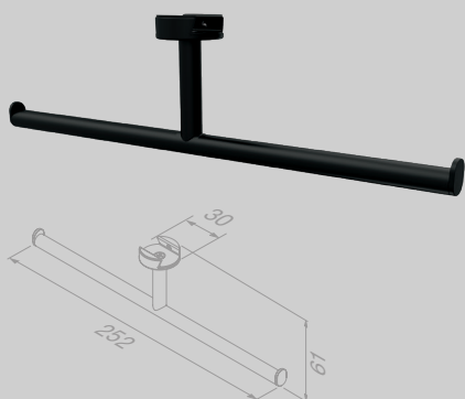
Toiletrolhouder zonder klep dubbel (Black) Toilet roll holder without cover double (Black) 918204-06
